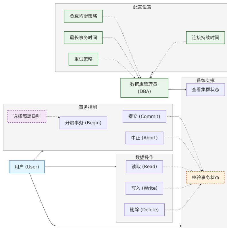
图 5-1 系统用例图
