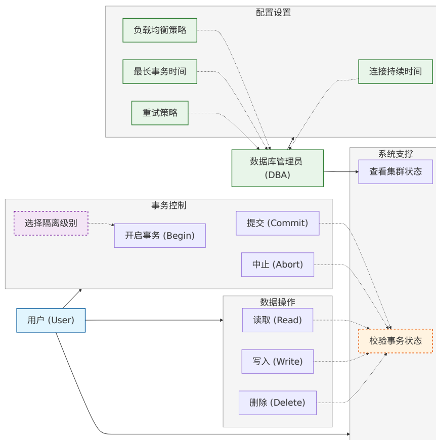
图 5-1 系统用例图
