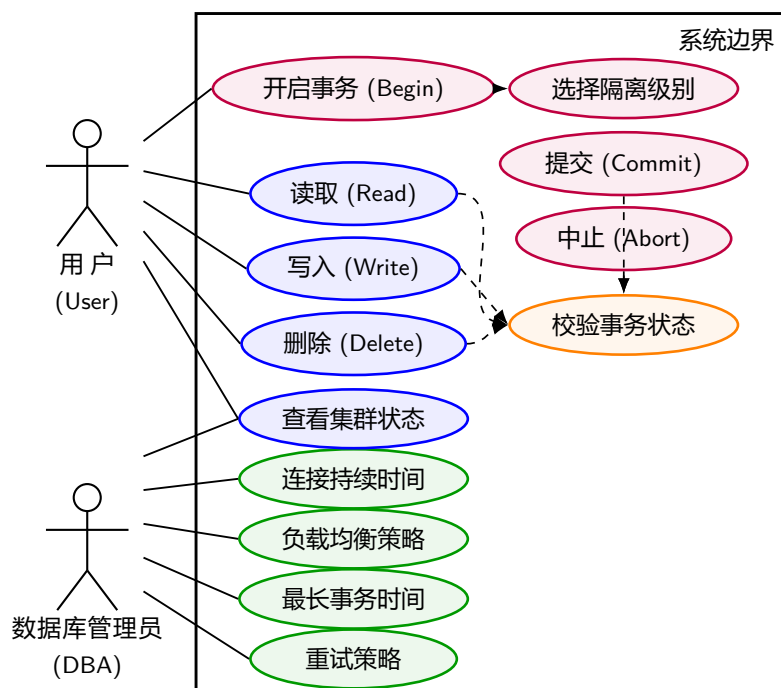
图 5-1 系统用例图
