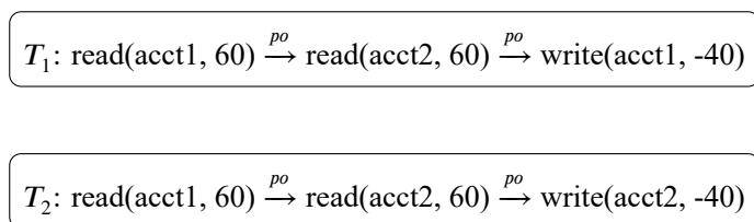
图 2-6 写偏斜示例
