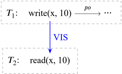
图 2-3 脏读示例
