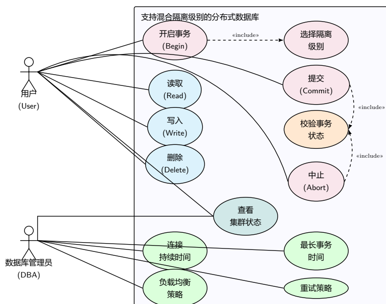
图 5-1 系统用例图
