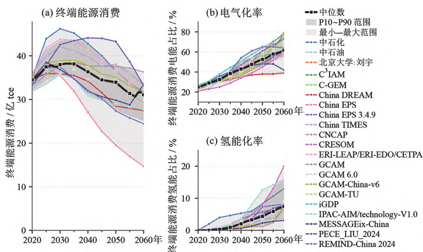
图 5 2020—2060 年中国终端能源消费 (a)、电气化率 (b) 和氢能化率 (c)
