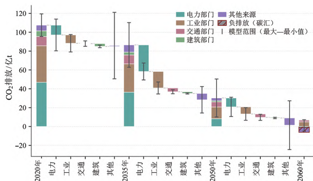
图3 不同时期各部门减排贡献
