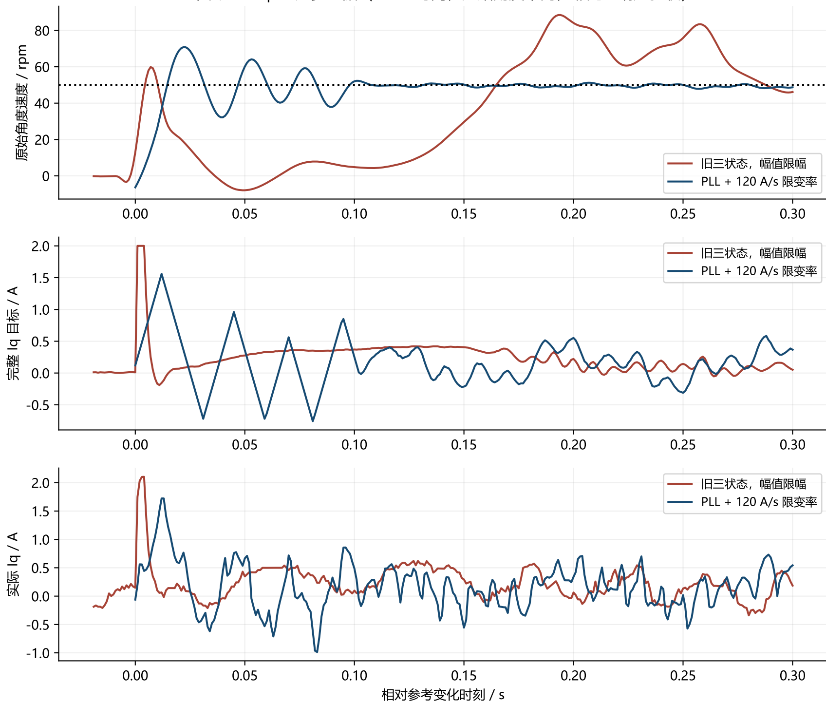
单次 +50 rpm 起步证据 (MCU 时间; 起始角度不同, 非完整响应验收)
