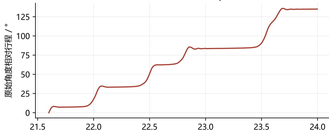
用户日志：目标 10 rpm
