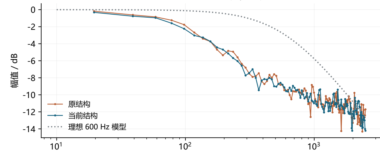
D 轴目标 → 同轴测得电流
