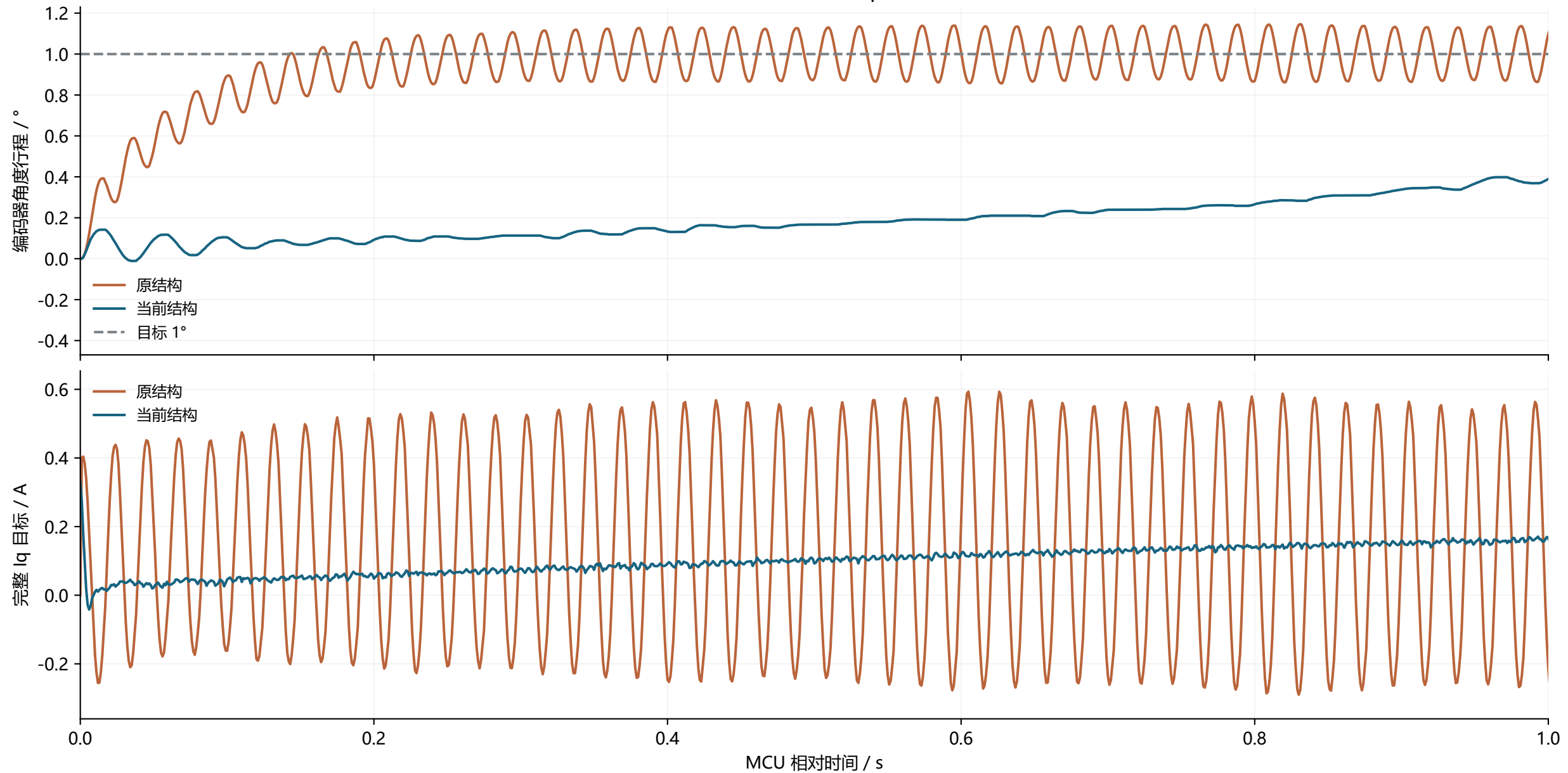
1° 位置小阶跃，位置 P=4 rpm/° 保持不变
