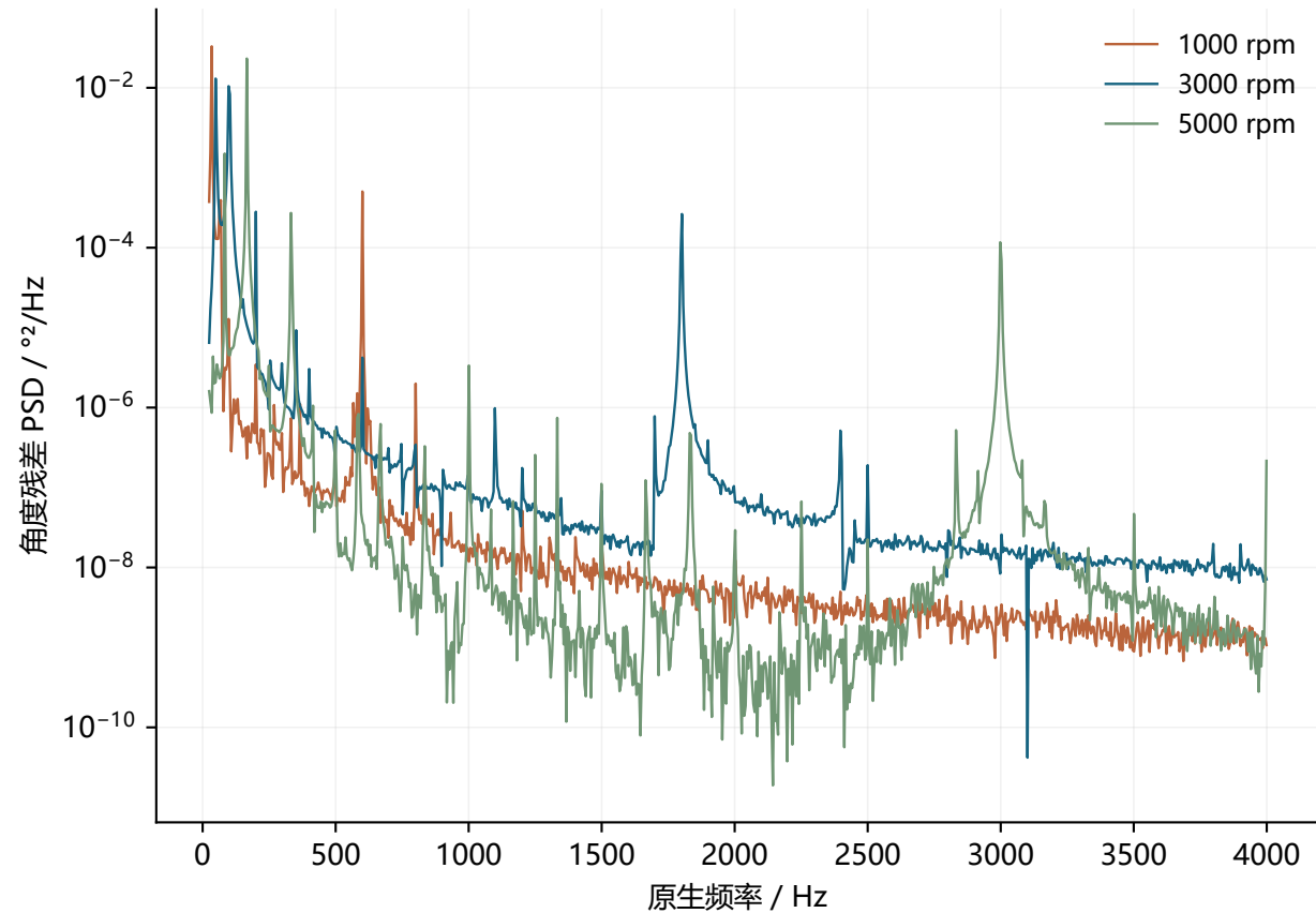
20 kHz 原生角度记录
