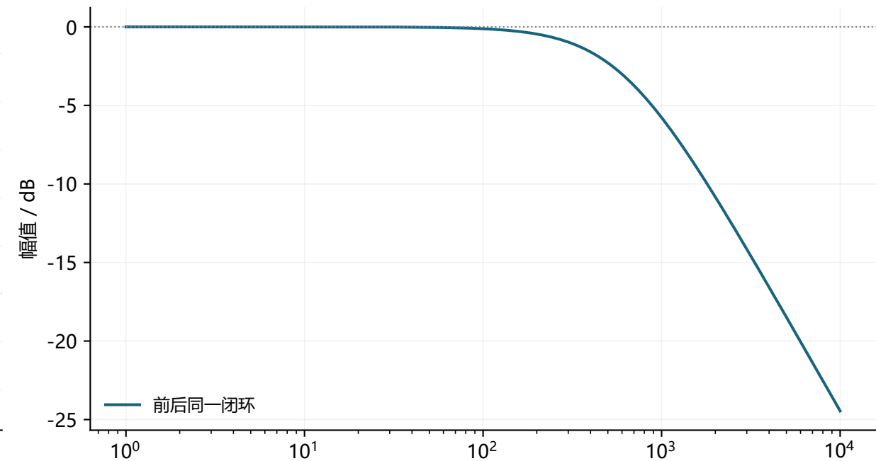
闭环目标 \rightarrow 测量电流
