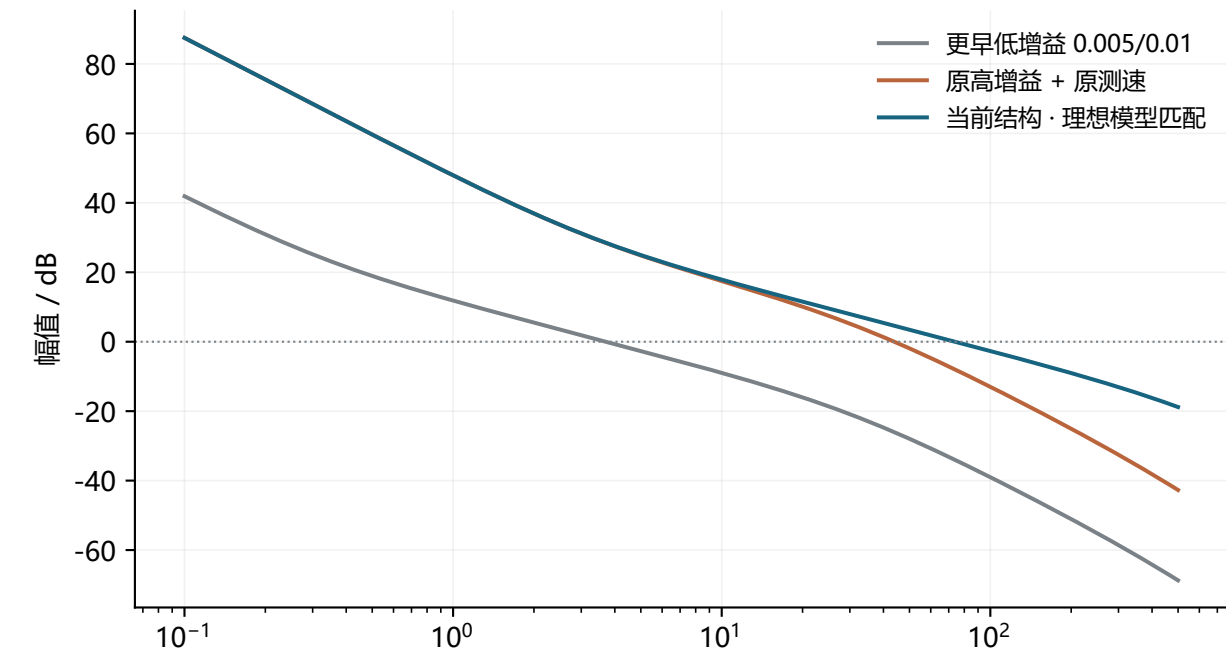
名义开环 · 0 dB 交越与相位
