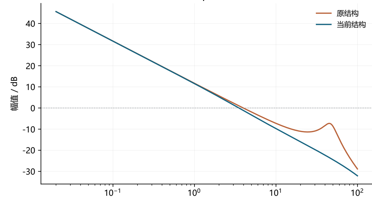
位置开环：6Kpos × T速度 / s
