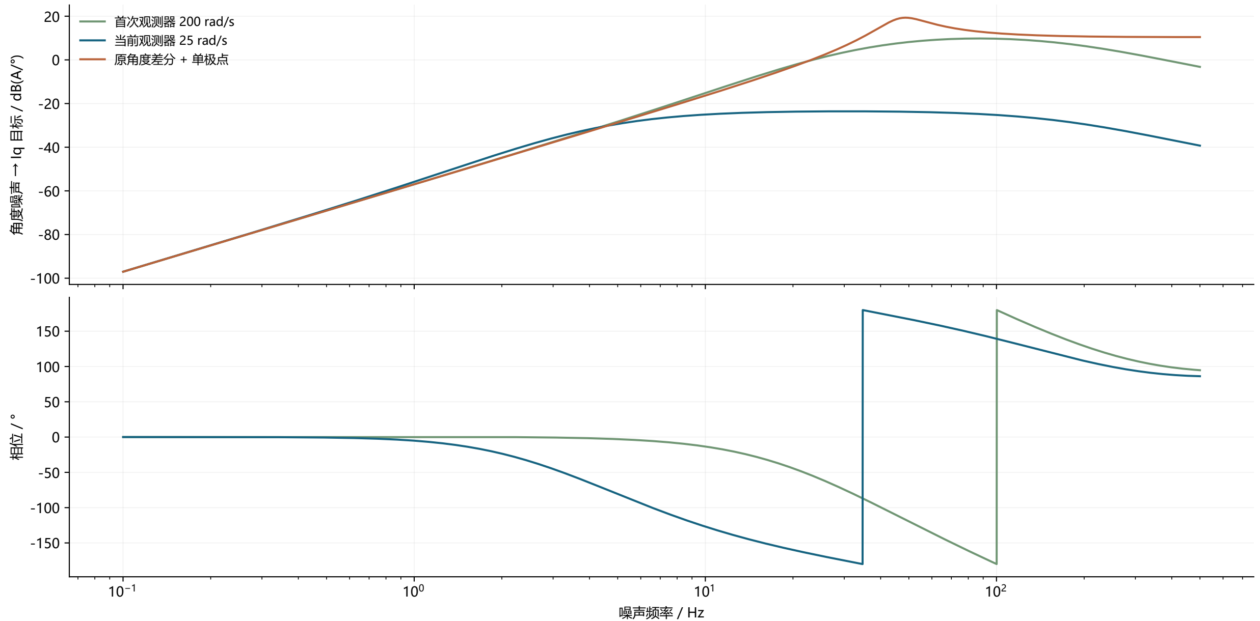
相同速度 PI 增益下的角度噪声传播
