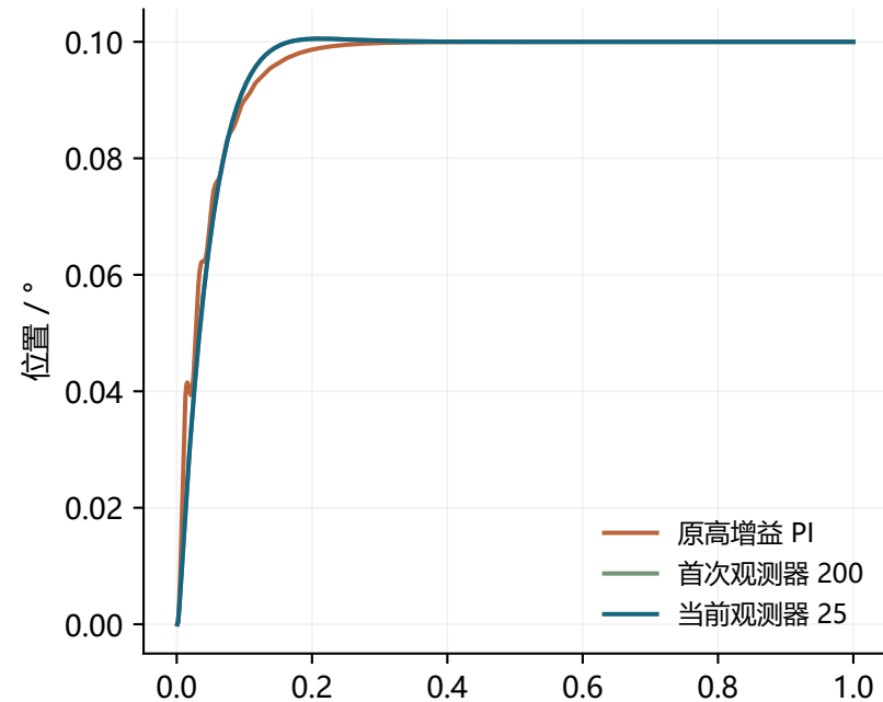
0.1° 位置小阶跃
