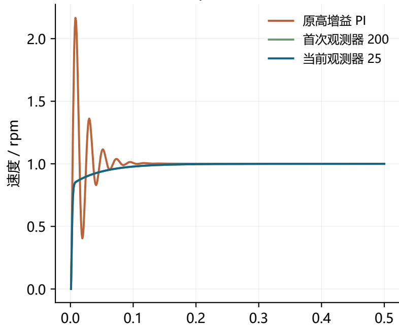
1 rpm 小阶跃
