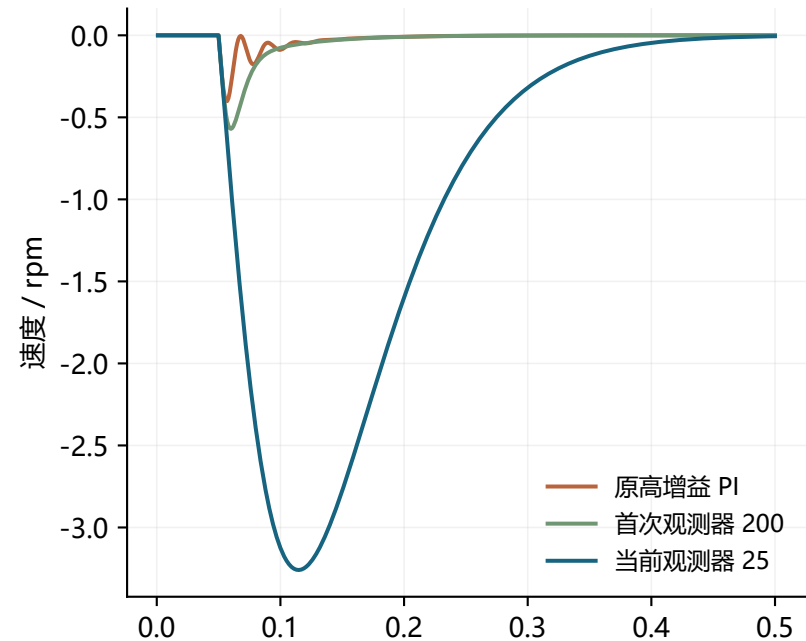
未知负载 +0.02 A 等效扰动
