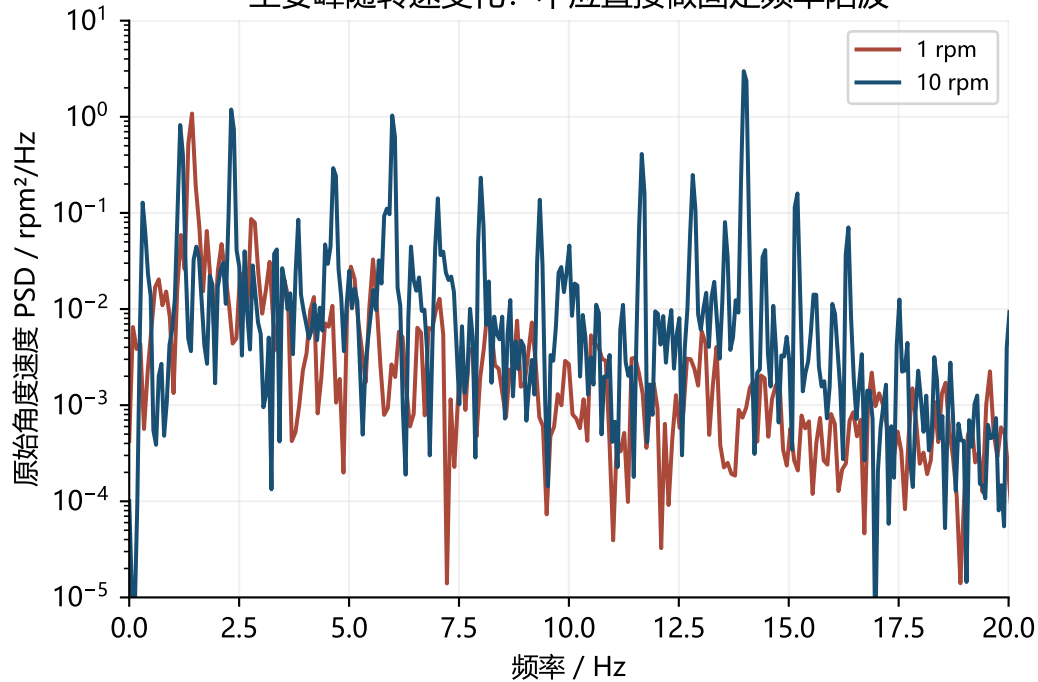
主要峰随转速变化：不应直接做固定频率陷波
