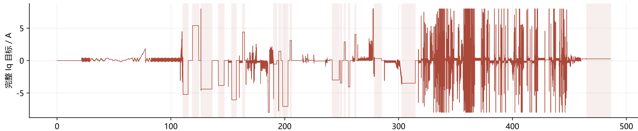
新协议段名义时间 / s (500 Hz, 无 MCU 时间戳)
