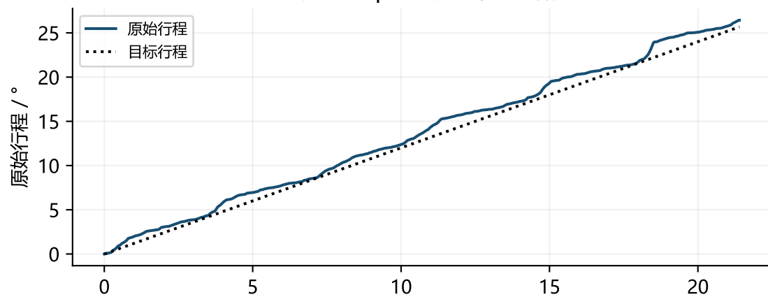
目标 0.2 rpm：完整稳态片段
