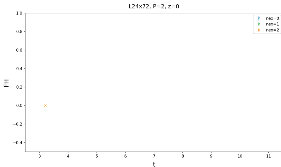
图 1: FH(t) 多 nex 对比 ( z=0 )。
