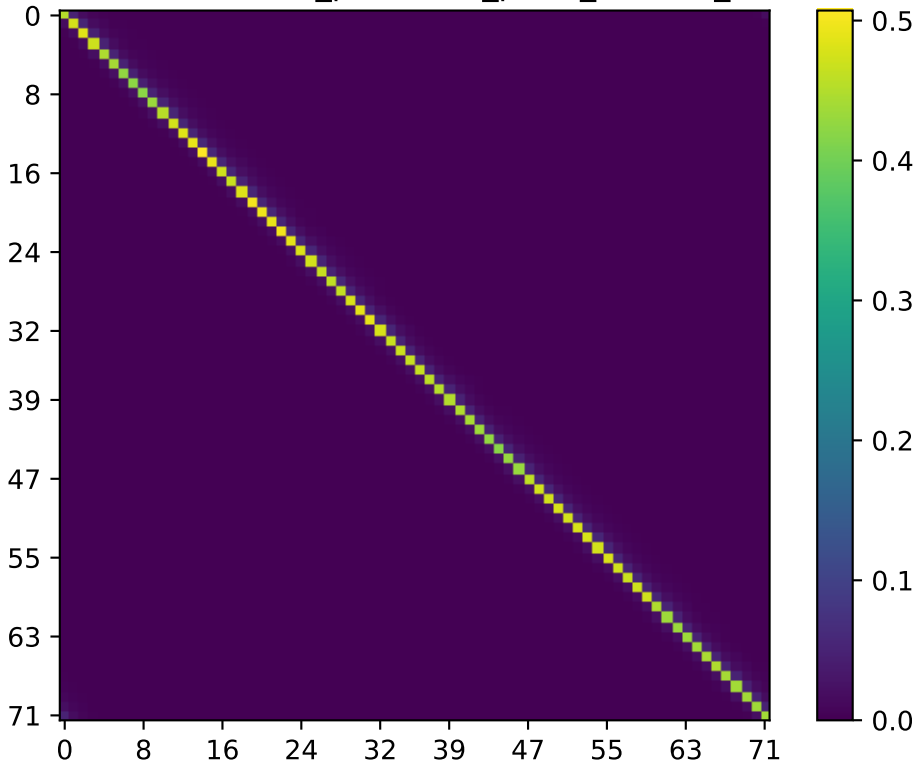
Real Part of two_point/two_point_L24x72_cc
