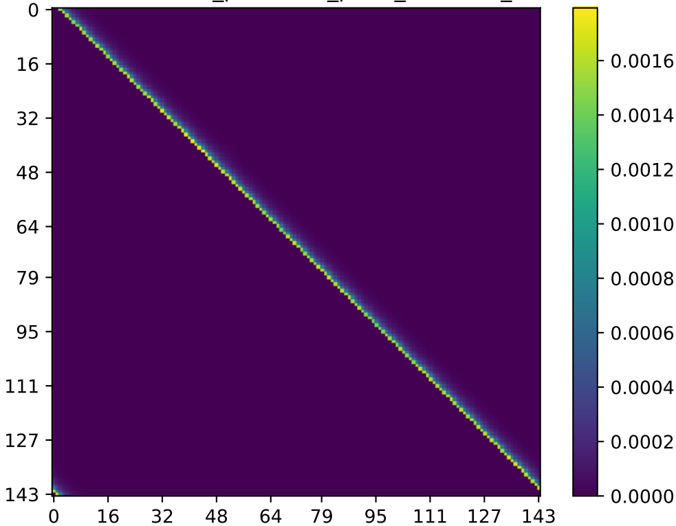
Real Part of two_point/two_point_L48x144_dhx
