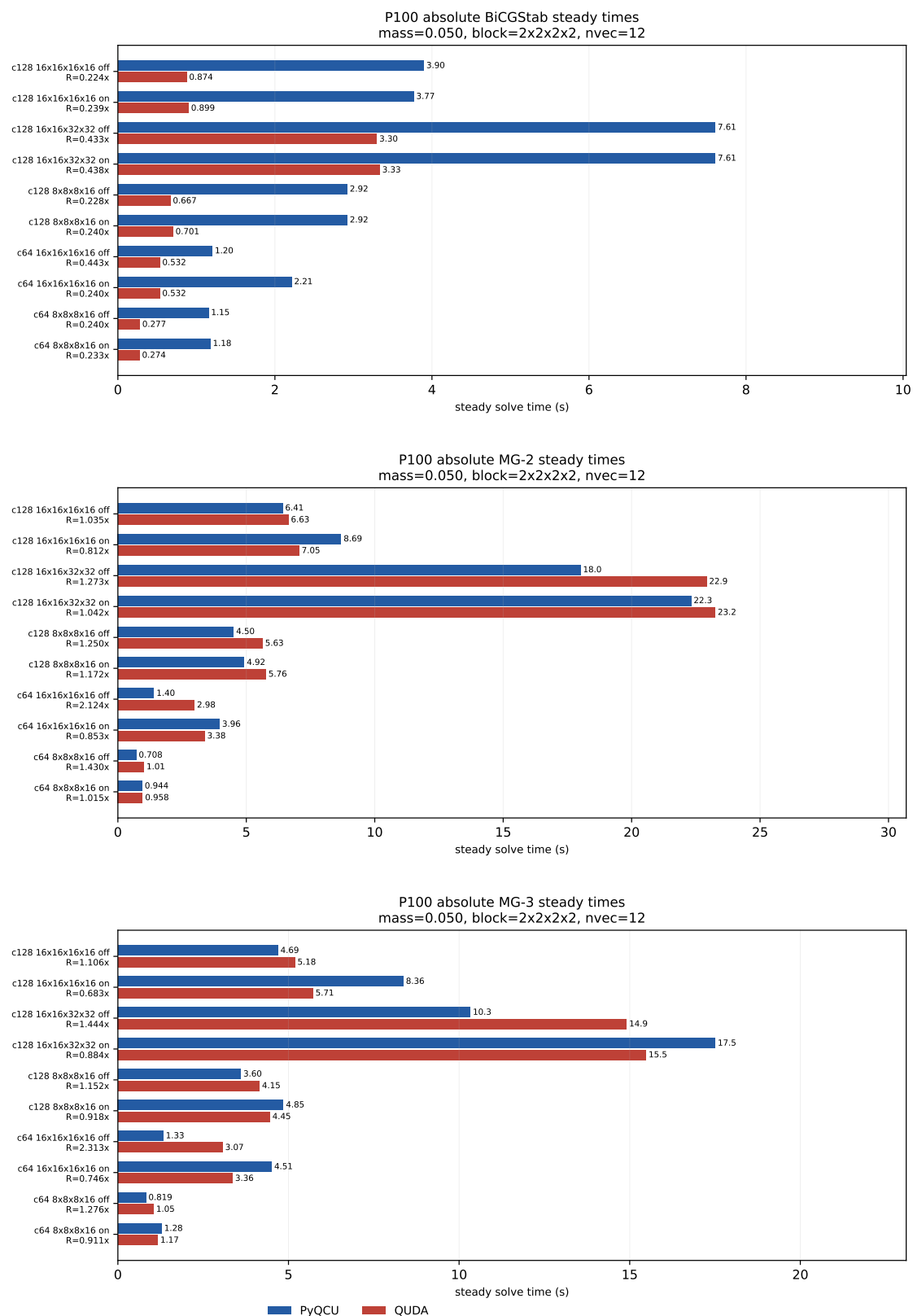
图 2: (续) P100 的 BiCGStab、MG-2、MG-3 绝对 steady 耗时。面板标题和条带标签采用与 V100 相同的字段口径。
