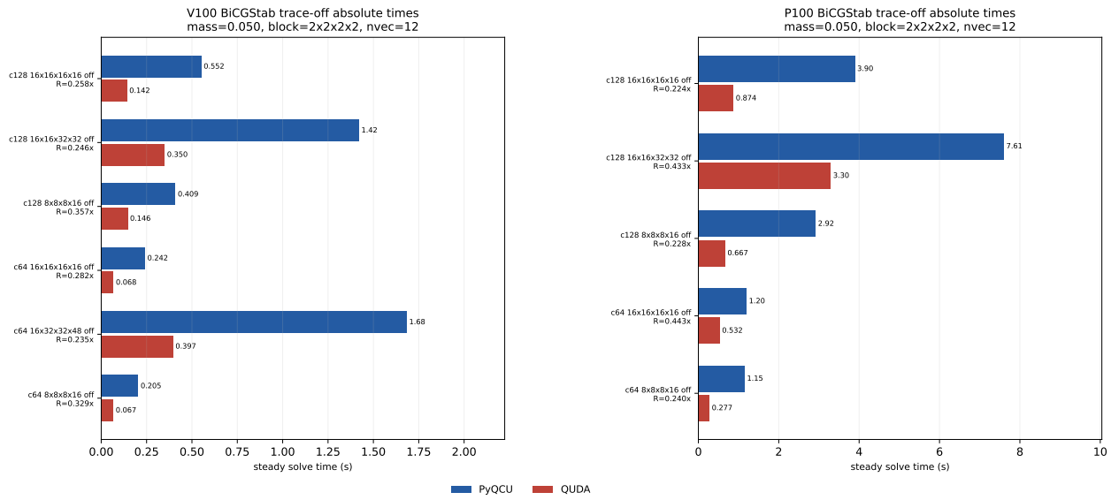
图 8: BiCGStab 参考的绝对 steady 耗时。每个条带标签保留格点、trace 与 R ；mass 只在面板标题中给出一次。
