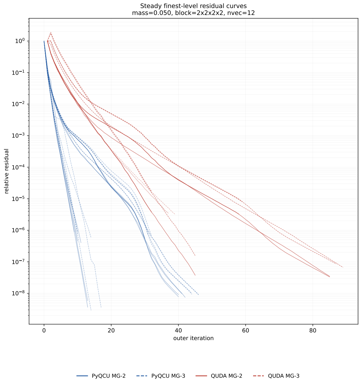
图 7: 最细层残差总览。44 条 side/case 曲线保留为细线, PyQCU/QUDA 与 MG-2/MG-3 使用四个分组标签; 纵轴为对数相对残差, 图例位于绘图区正下方。
