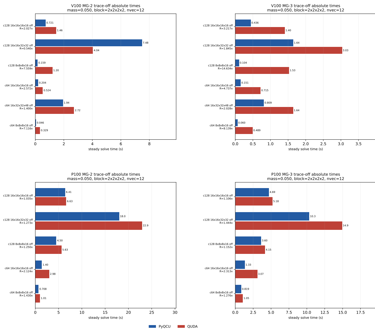
图 3: trace-off MultiGrid 的绝对 steady 耗时。四个面板分别对应 V100/P100 与 MG-2/MG-3; 比值放在左侧标签, 不进入绘图区。
