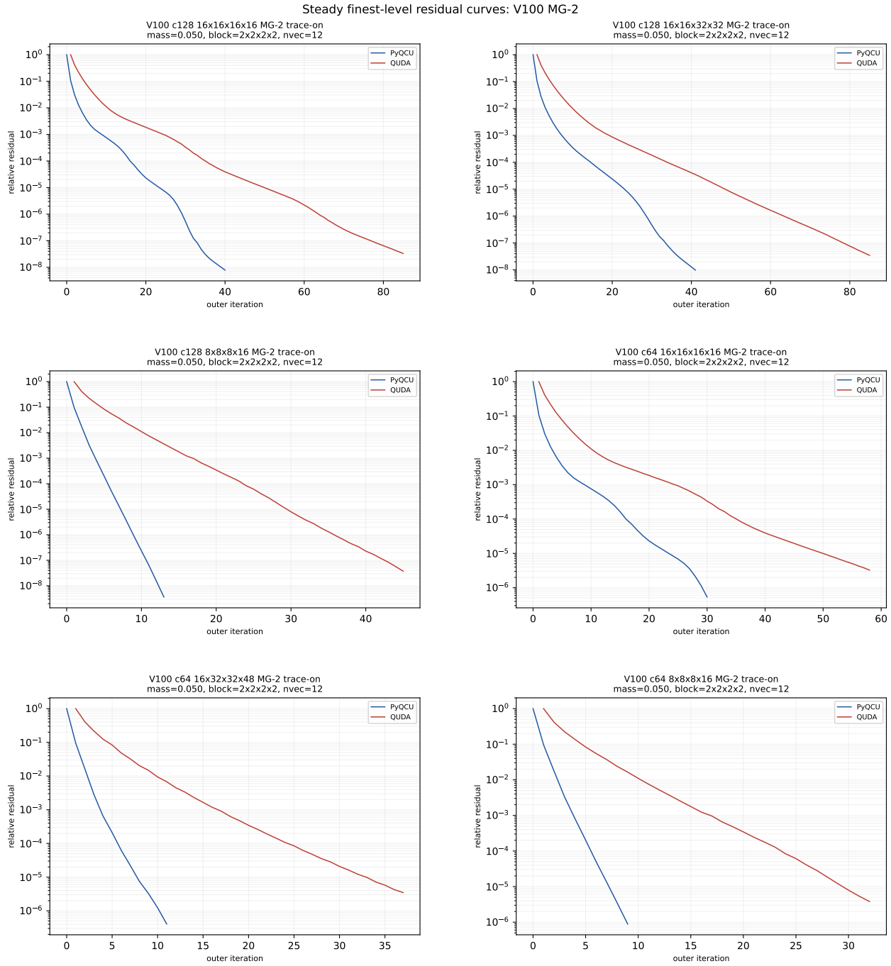
图 6: 最细层残差小面板 (V100 MG-2)。纵轴为相对残差对数轴, 横轴为线性 outer iteration; 图内保留 mass、block 和 nvec。该图从原图 6 拆成四页, 避免 12 个以上子图挤在一页。
