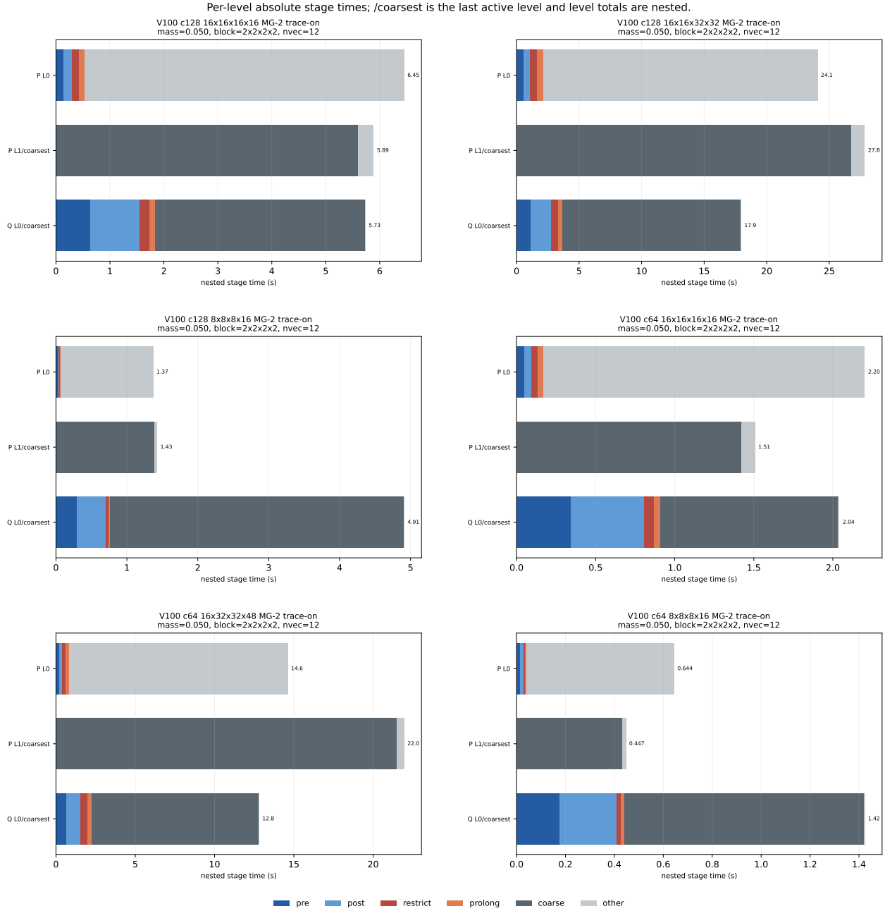
图 4: 逐层绝对阶段耗时: V100 MG-2。P/Q 分别表示 PyQCU/QUDA, /coarsest 表示最后有效层; 图内保留 mass、block 和 nvec。
