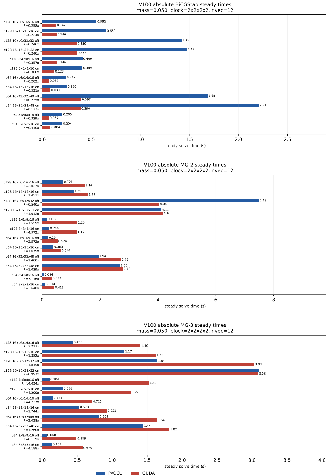
图 2: V100 的 BiCGStab、MG-2、MG-3 绝对 steady 耗时。每个面板标题保留 mass、block 和 nvec；条带标签只保留格点、精度、trace 与 R。
