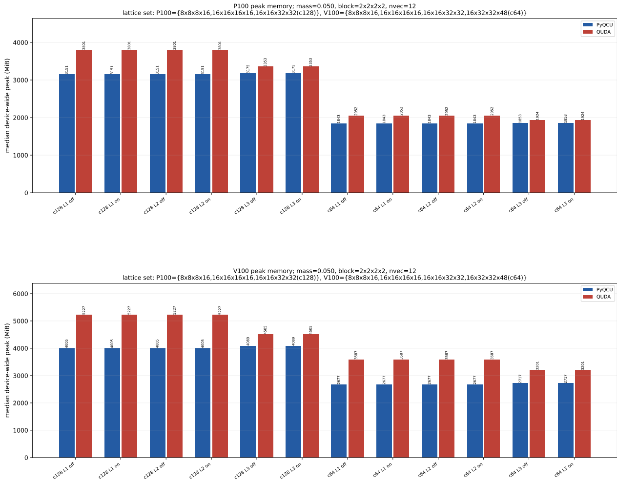
图 5: 设备级峰值显存按设备、精度、MG 层数和 trace 模式的中位数。图内保留 mass、block、nvec 和 lattice set，不在标题重复 kappa。
