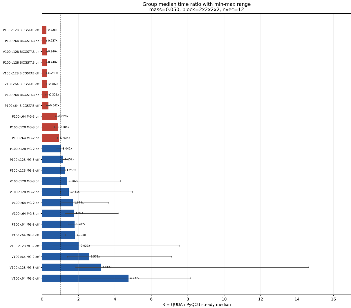
图 1: 分组中位时间比与组内 min-max 范围。横轴为 R = t_{\text{QUDA,steady}}/t_{\text{PyQCU,steady}} , 虚线为 R = 1 ; 图内保留 mass、block 和 nvec, 不在标题重复 kappa。
