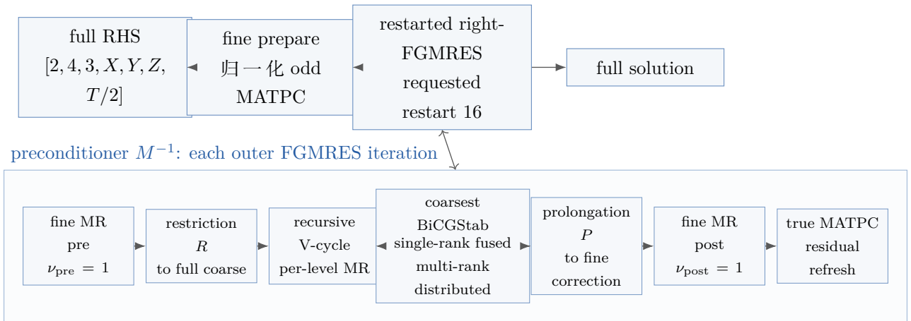
图 2: PyQCU test27 Strict-MG 的算法流水。蓝色框是实现路径，箭头表示数据依赖；最粗层为双分支：单 rank 可走 fused cooperative kernel，多 rank 走 host-driven distributed fallback。每个 restart 均回到同一个持久 hierarchy。
