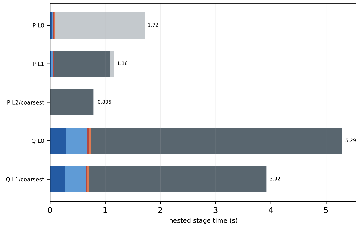
V100 c128 8x8x8x16 MG-3 trace-on
