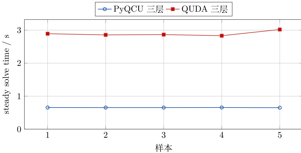
图 1: 正式大格 c64 五次 steady solve; 数据来自项目数据目录中的正式 JSON。
