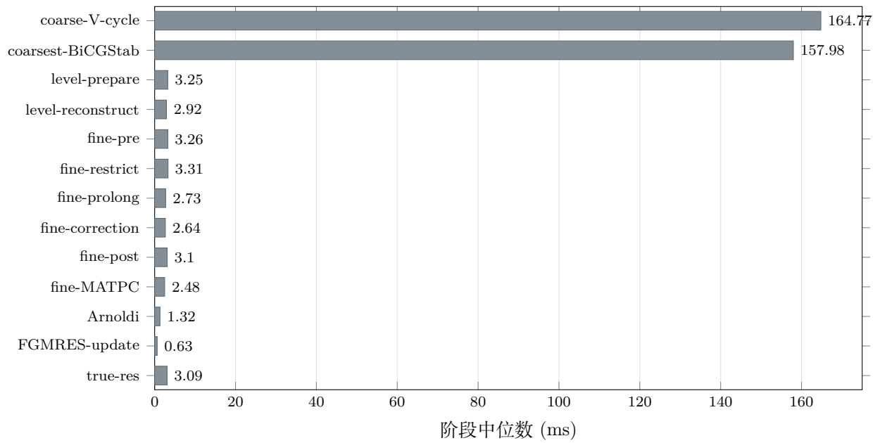
图 3: PyQCU Strict 阶段诊断。嵌套 stage 不可相加; coarse-V-cycle 内含 coarsest-BiCGStab, 且所有 stage 均含 trace 同步开销。
