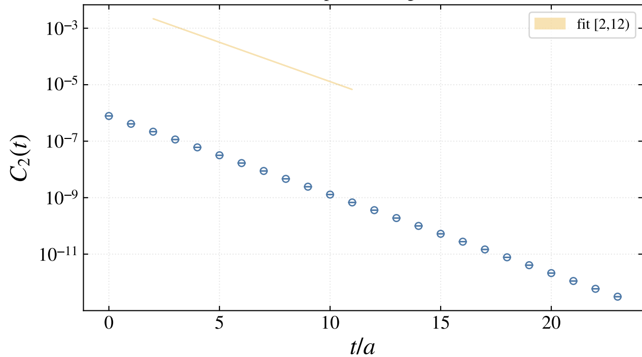
Proton 2pt (lamet-agent fit)
