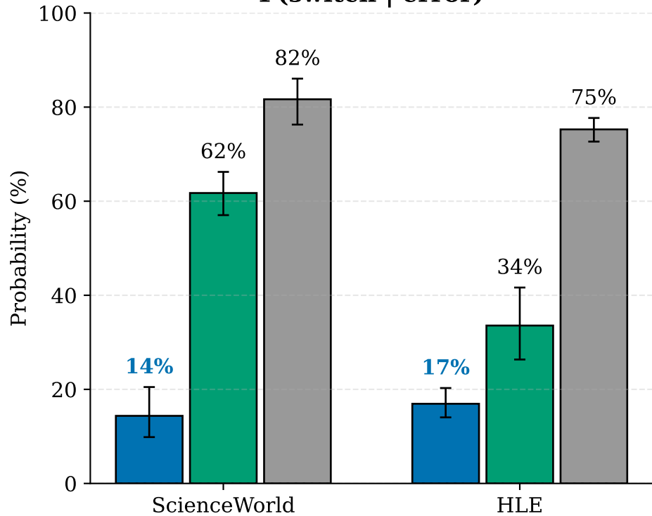
P(switch | error)
