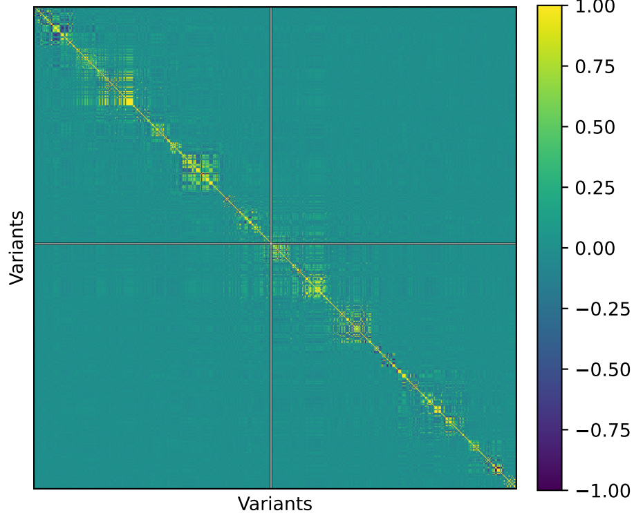
chr17:13528059:G:A — R (n=2984)
