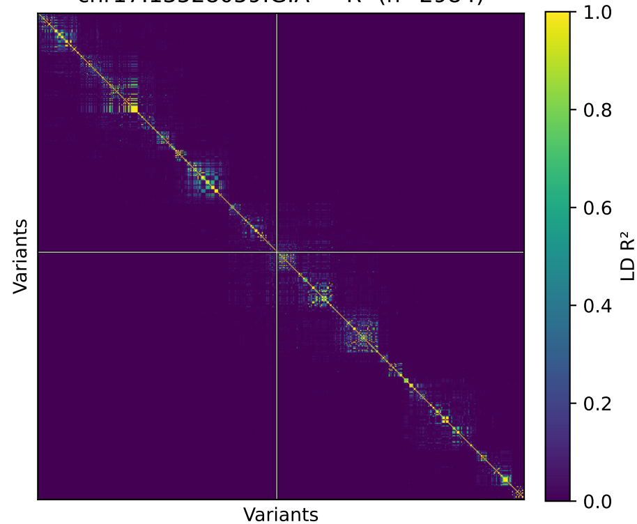
chr17:13528059:G:A — R^2 (n=2984)
