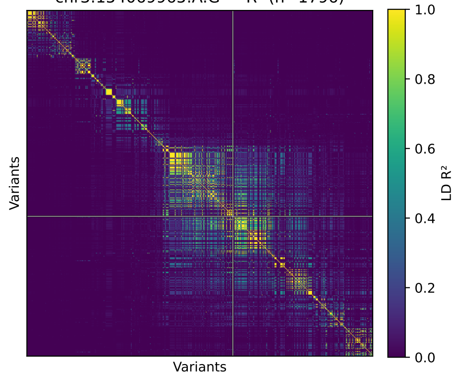
chr3:154069965:A:G — R^2 (n=1796)
