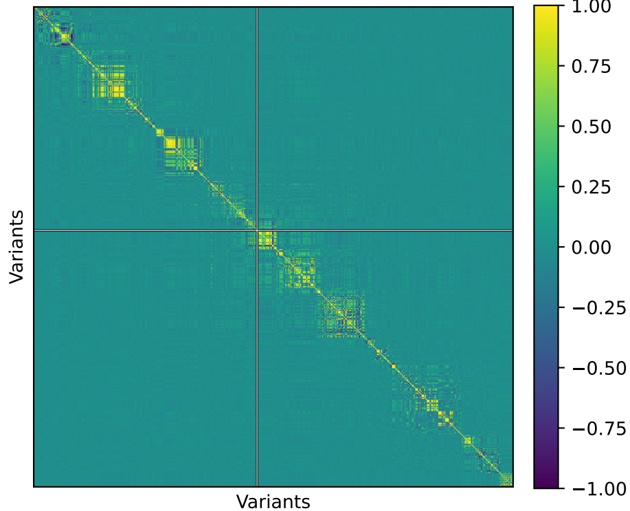
chr17:13528059:G:A — R (n=3135)
