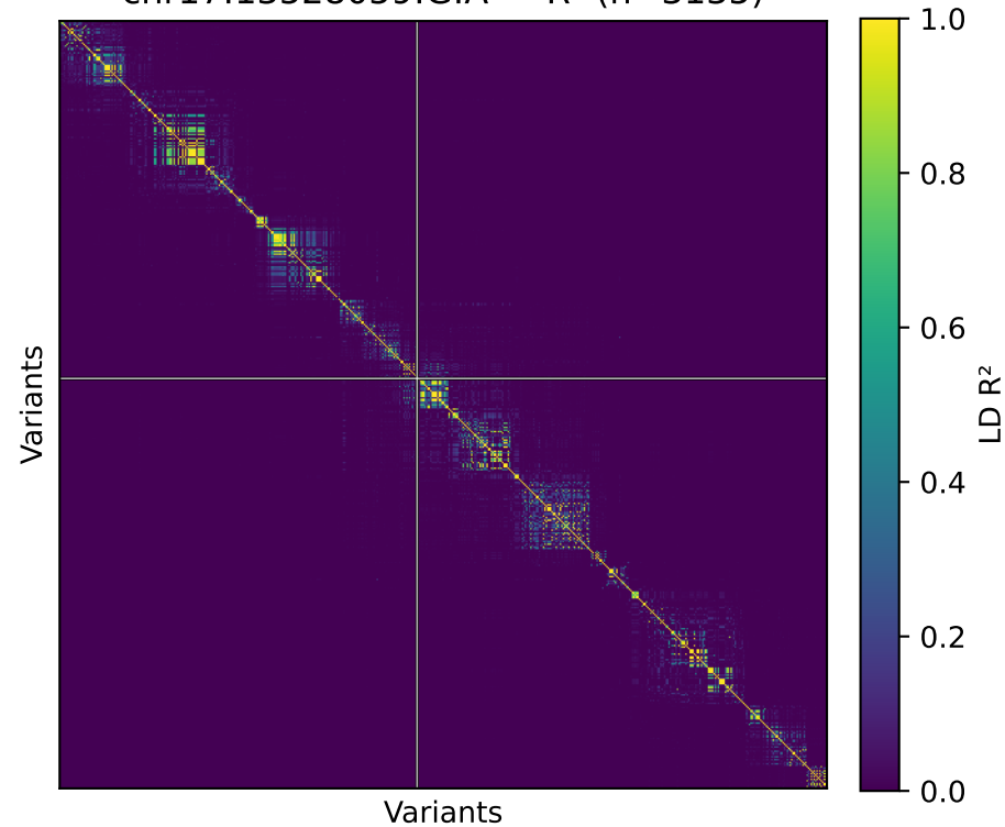
chr17:13528059:G:A — R 2 (n=3135)
