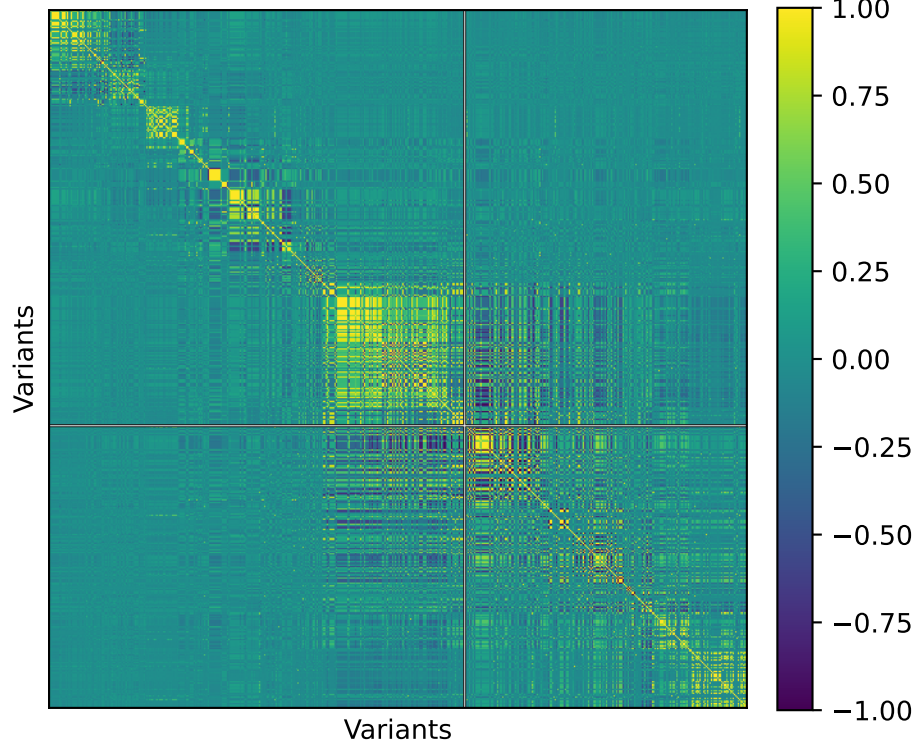
chr3:154069965:A:G — R (n=1796)
