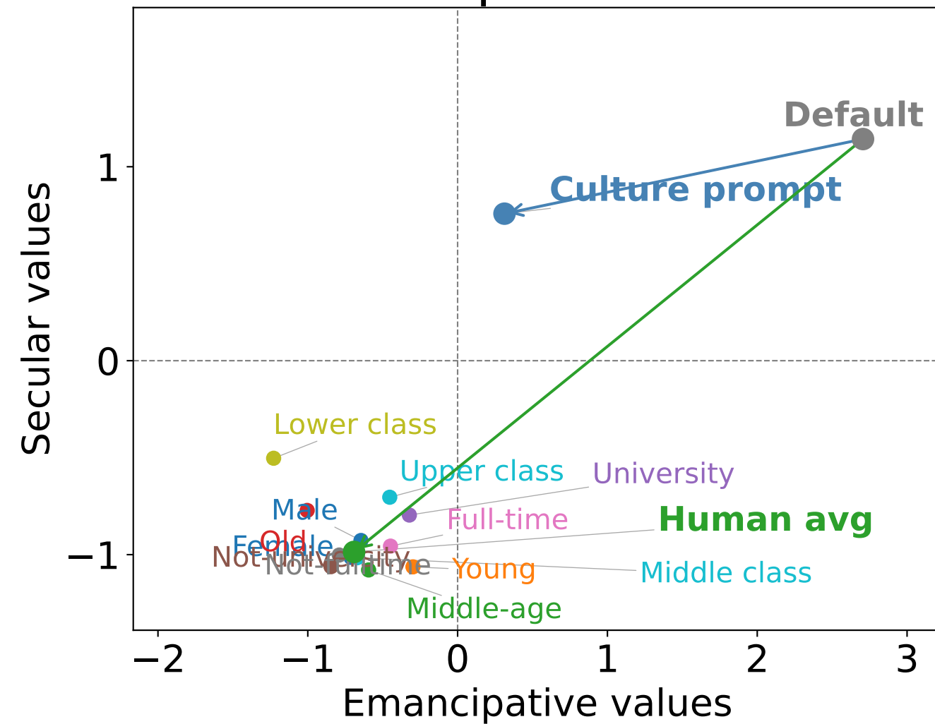
GPT | Armenia
