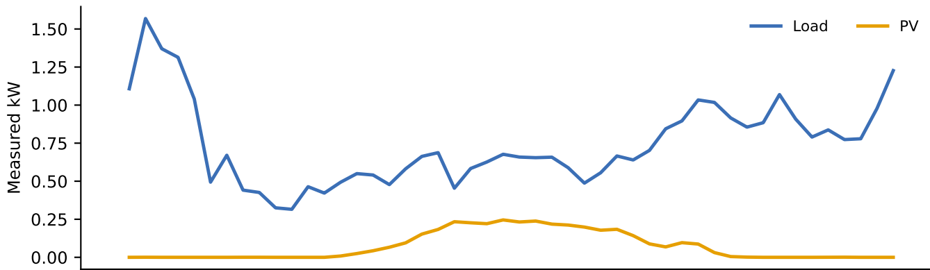
Ausgrid interval trajectory (2010-10-09)
