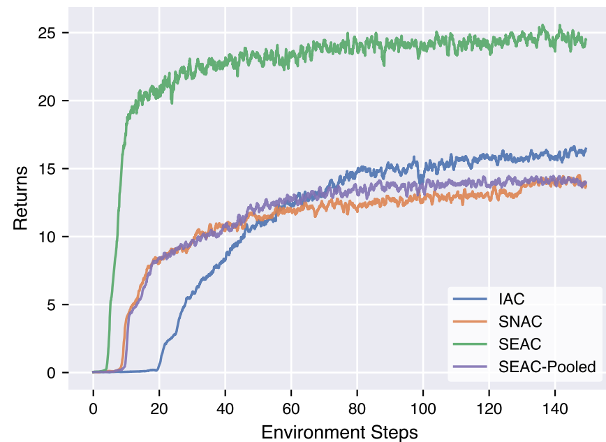
(d) small-4ag: Train Reward
