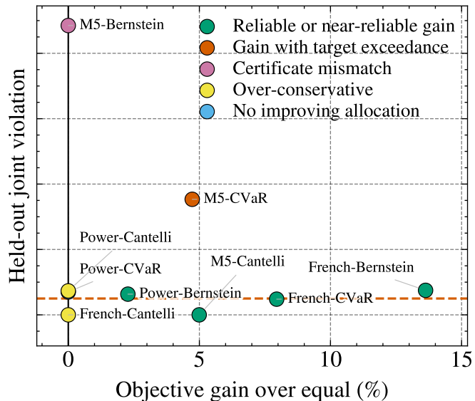
OOD
