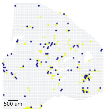
SpaGCN-style
