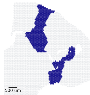
Spatial Leiden
