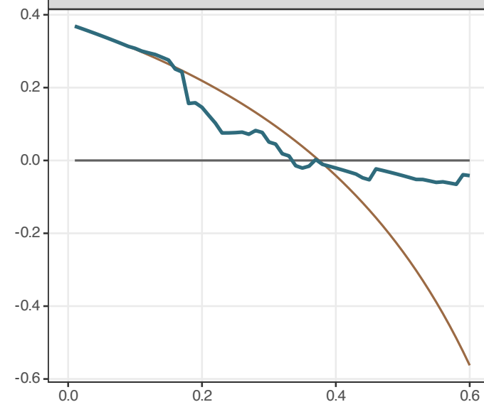
GSE76427
