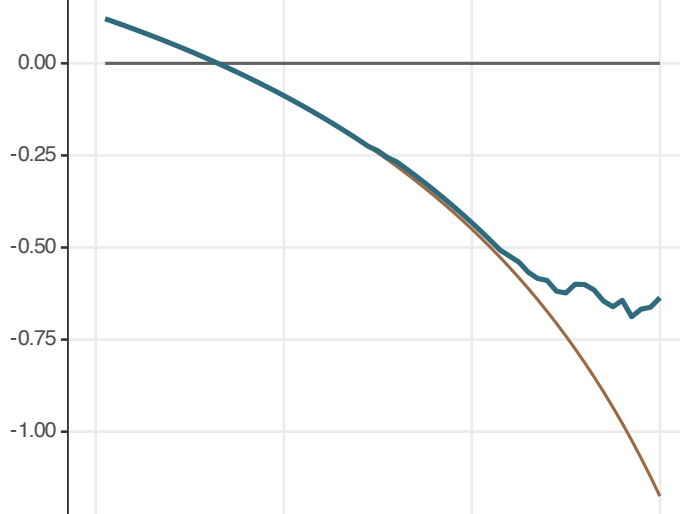
GSE76427
