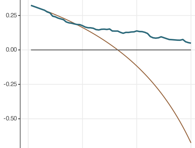
ICGC-LIRI-JP (HCCDB18)
