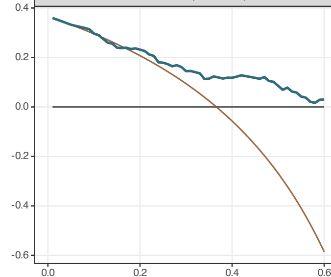
ICGC-LIRI-JP (HCCDB18)
