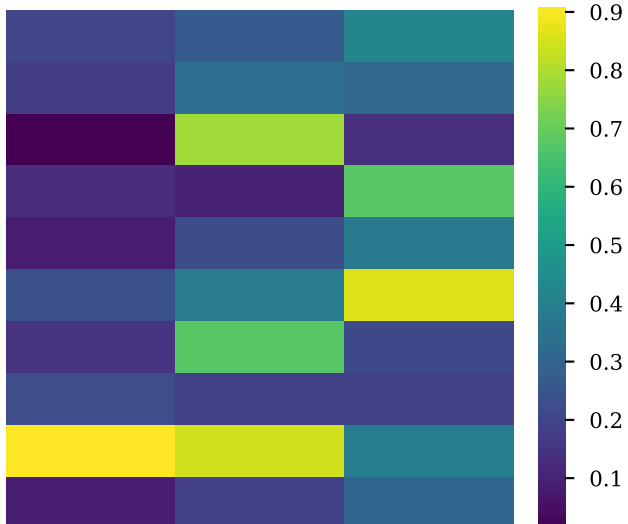
True \Lambda
