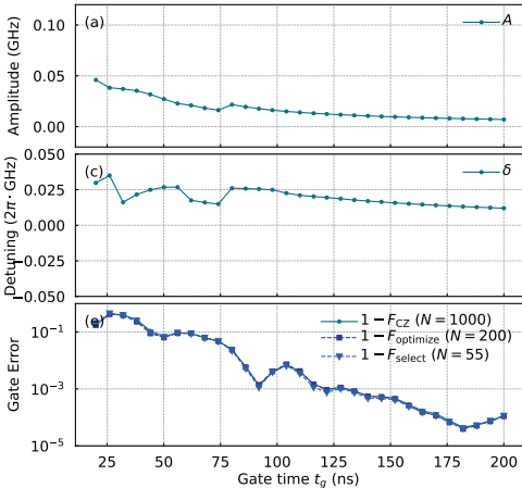
CZ Gate
