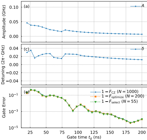
CZ Gate
