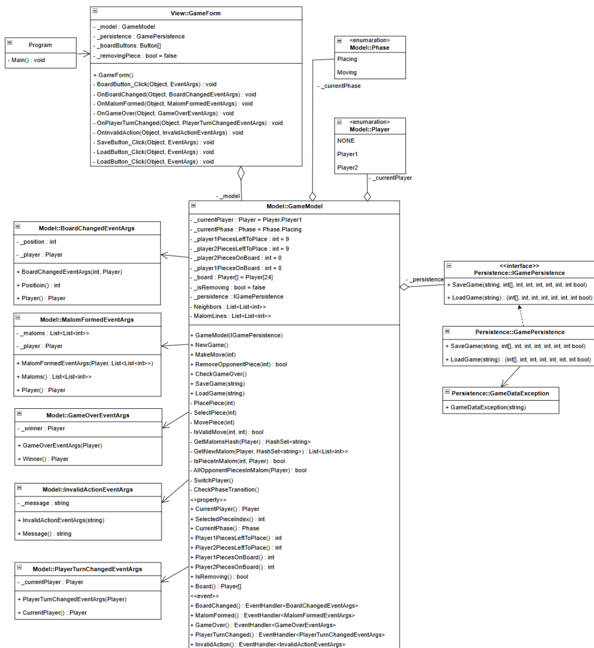
3. ábra: Az alkalmazás osztálydiagramja
