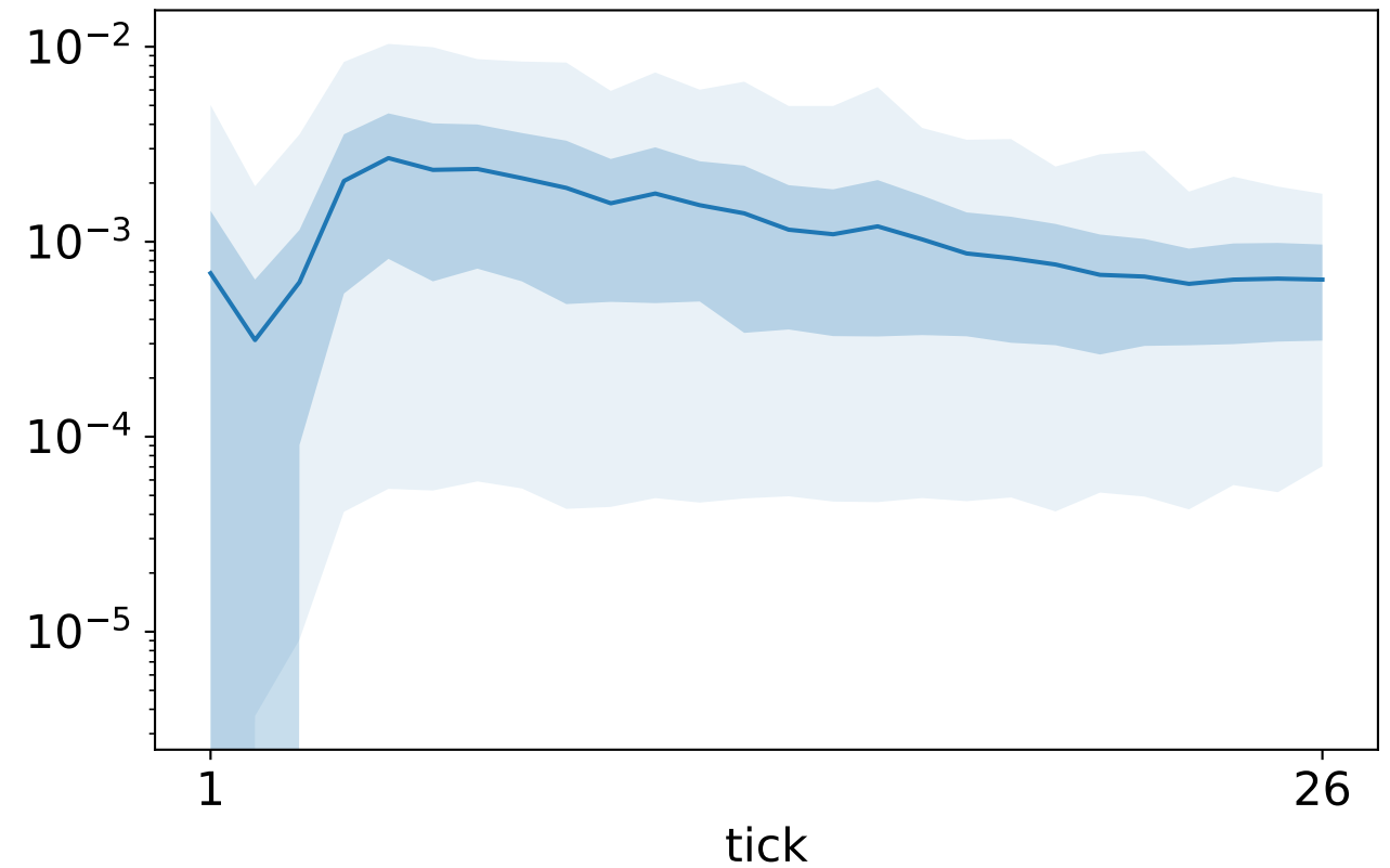
Gradient norm
