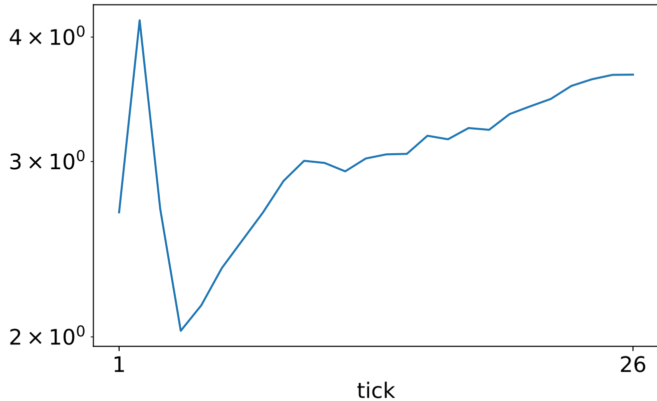
Parameter norm
