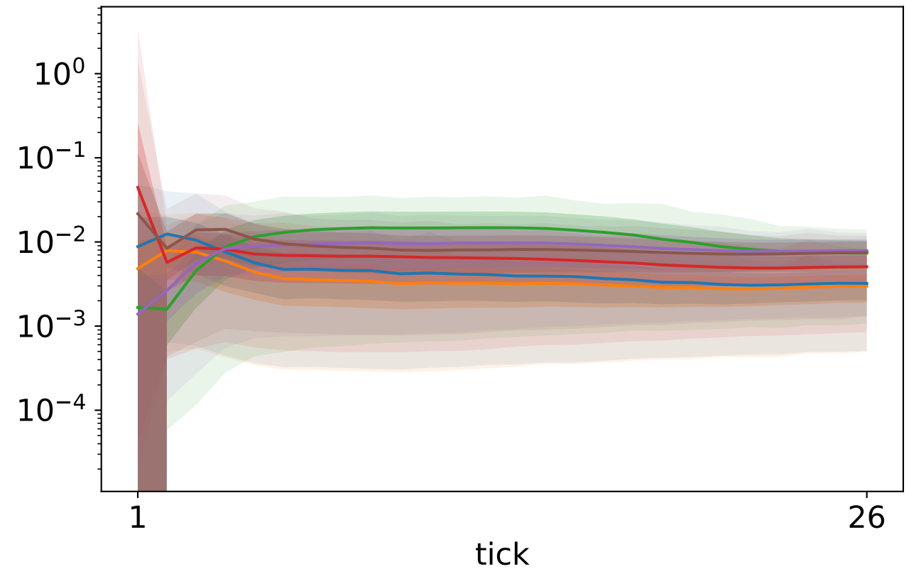
Gradient norm
