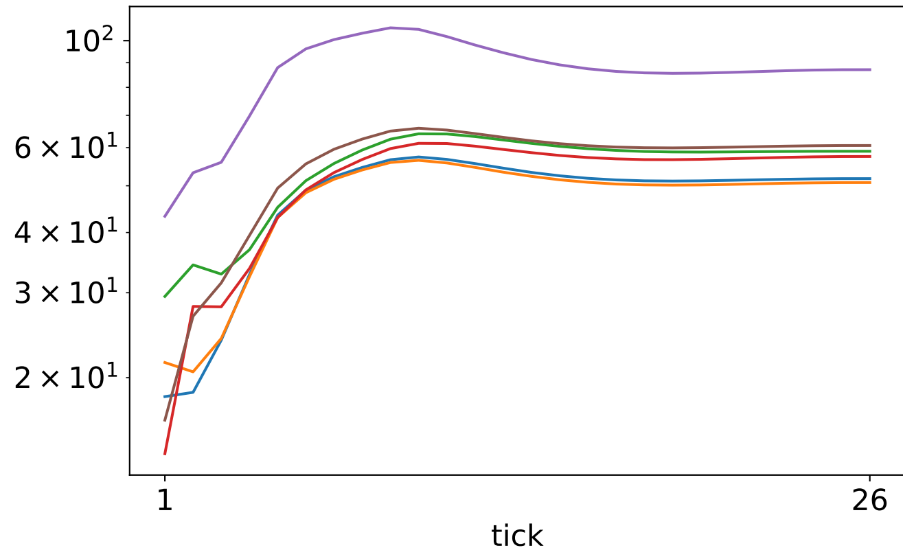
Parameter norm
