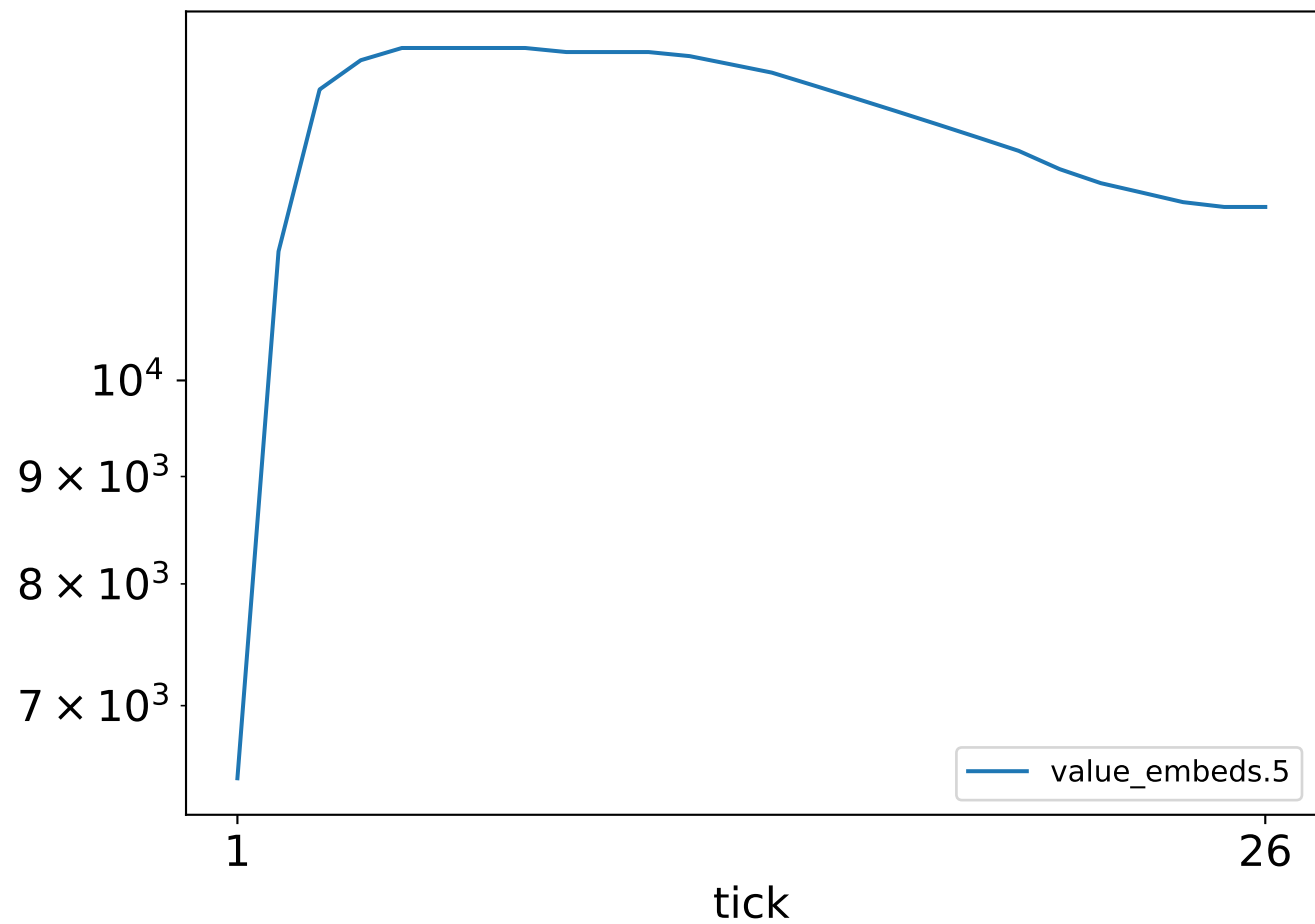
Parameter norm
