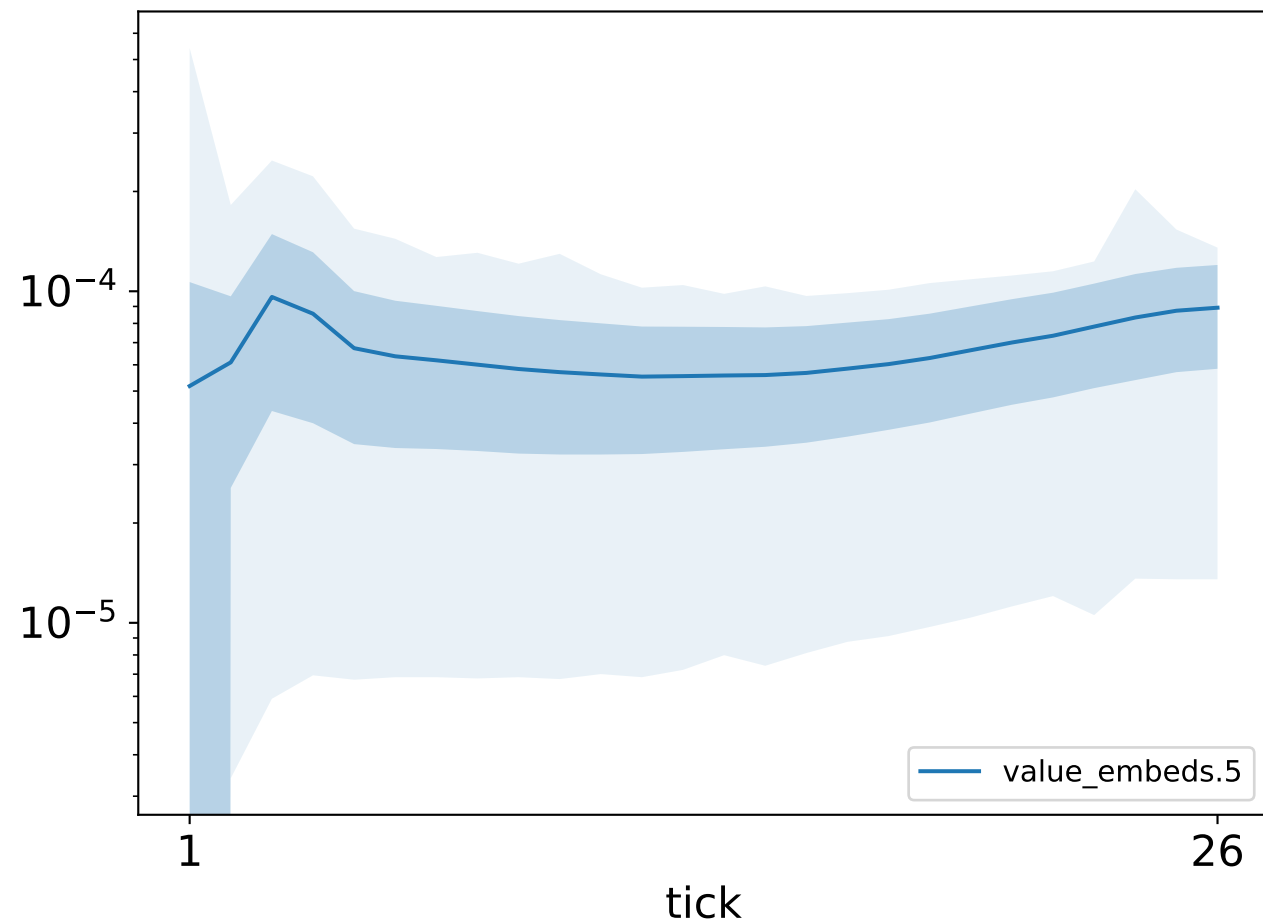
Gradient norm
