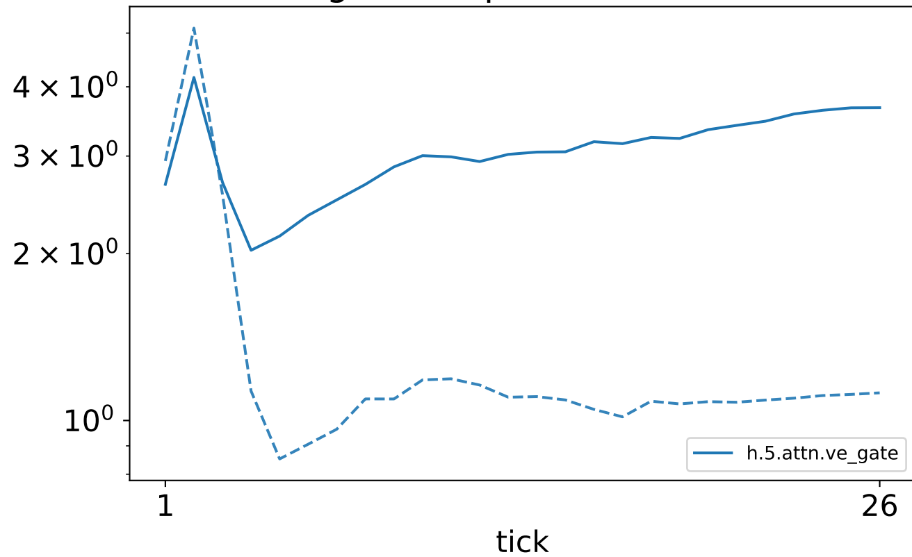
VE gates — parameter norm
