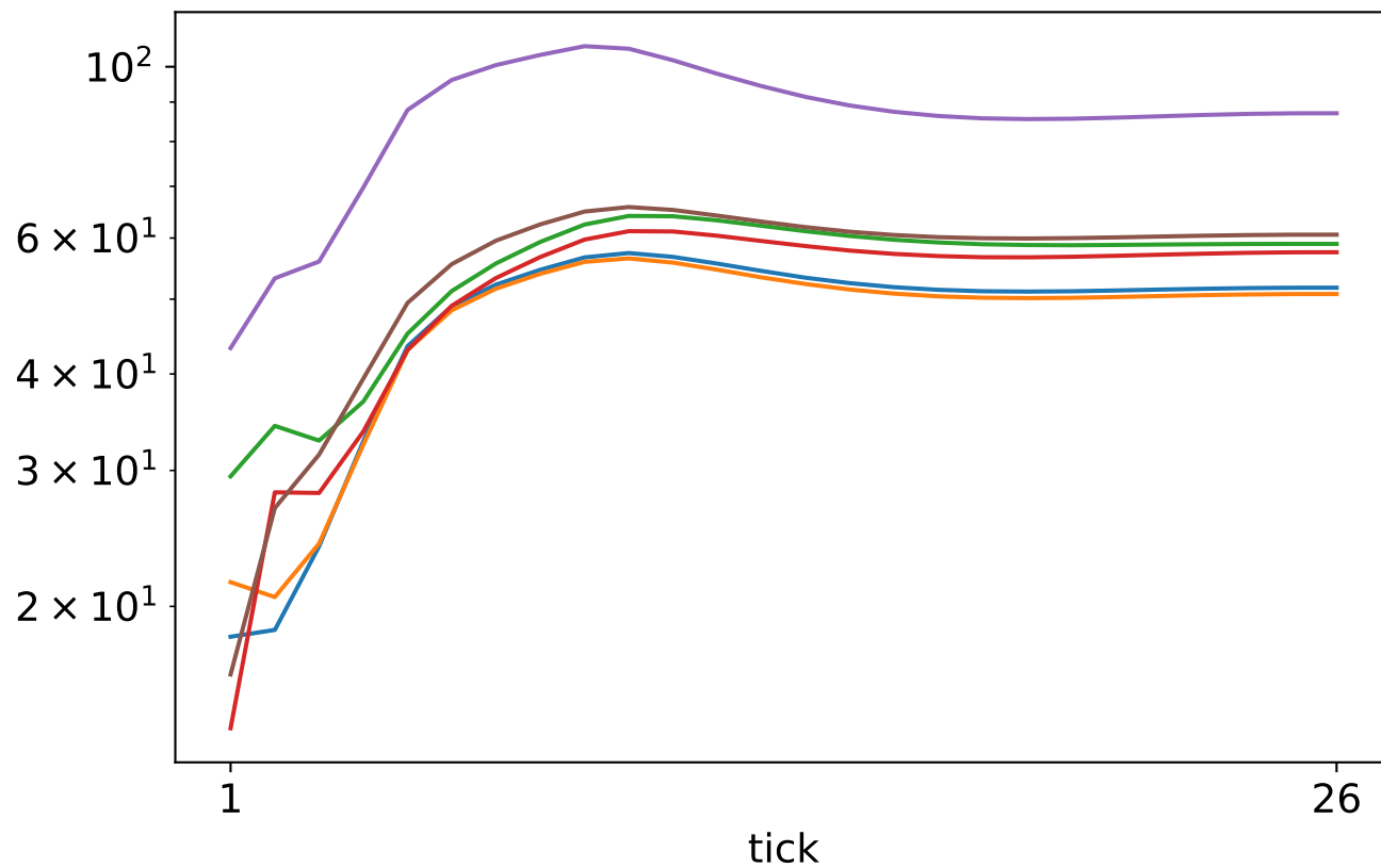
Parameter norm
