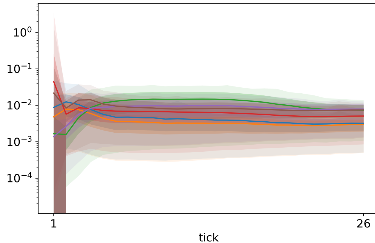
Gradient norm
