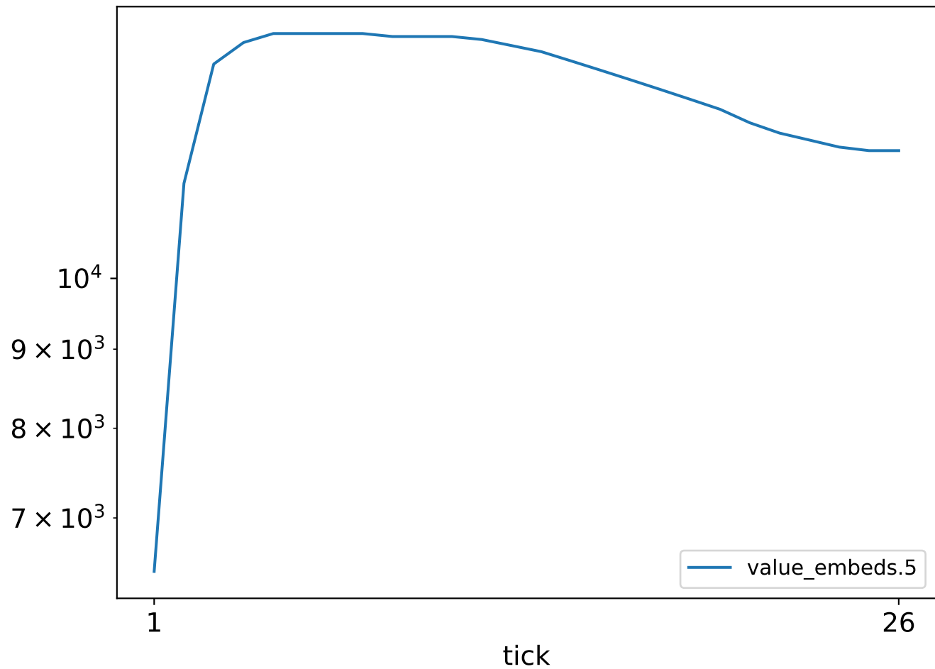
Parameter norm
