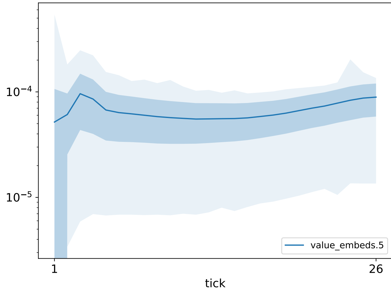
Gradient norm
