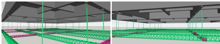
二层展厅母架示意图
