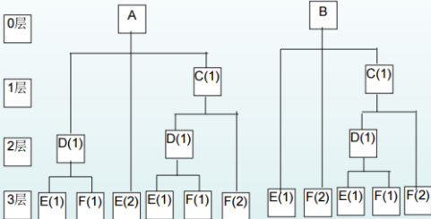
图1 电表A、B的物料清单
