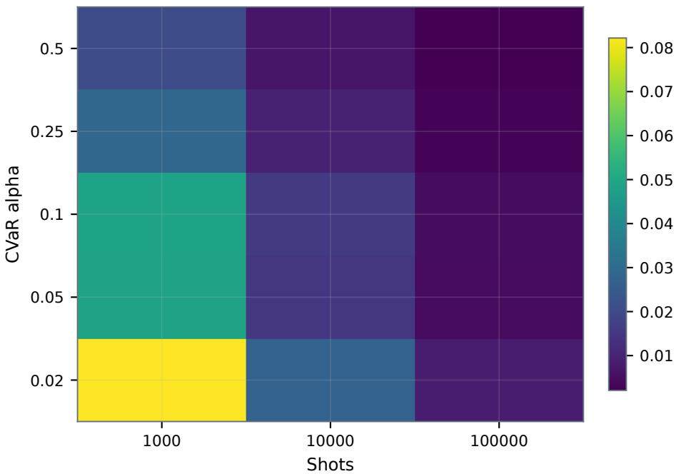
a CVaR estimator RMSE
