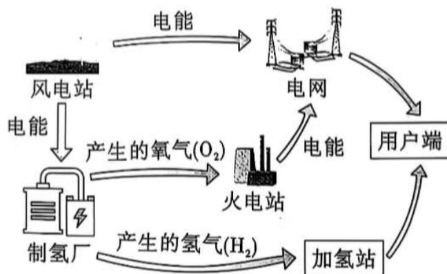
“碳—氢—风—电”能源耦合模型
